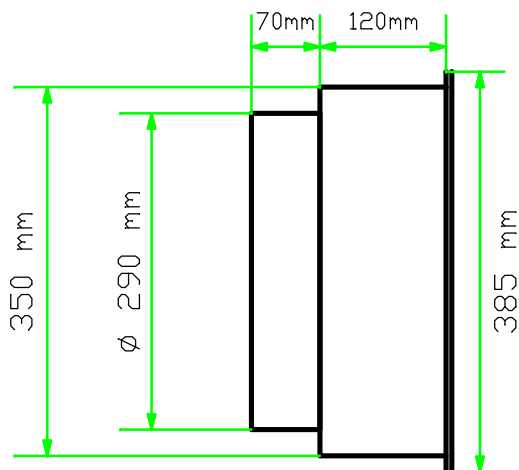
Unità di pressurizzazione EV300
