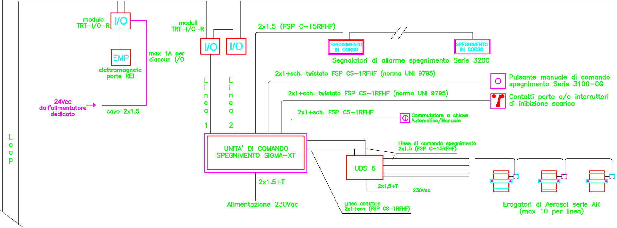
Schema esemplificativo di loop TRIDENT con comando per spegnimento ad Aerosol
