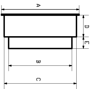
Vista laterale unità di pressurizzazione
