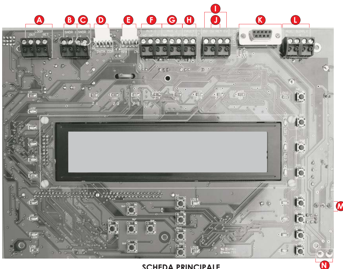
SCHEDA PRINCIPALE
