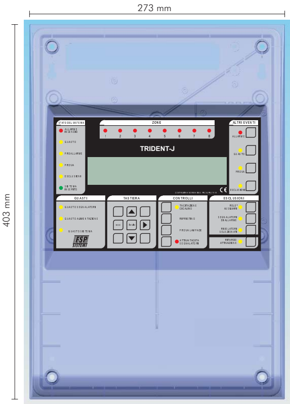
VISTA FRONTALE
