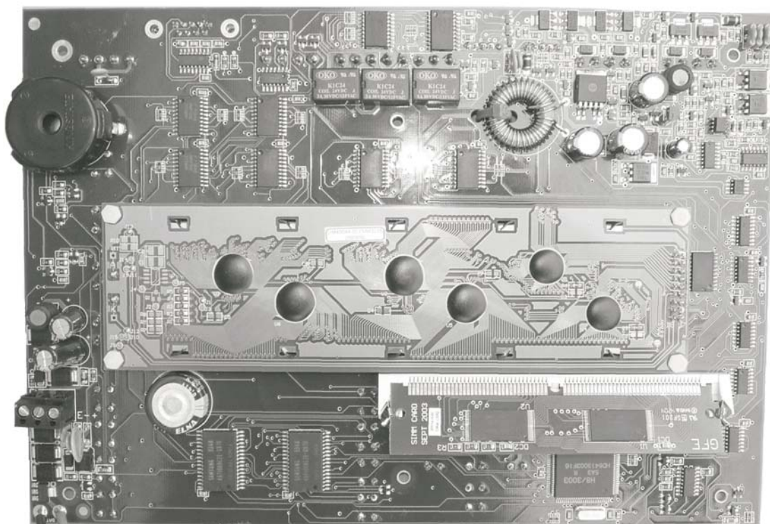
VISTA POSTERIORE
