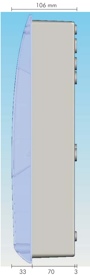
VISTA LATERALE
